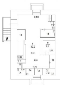
Подвал - 93,8 кв.м.
