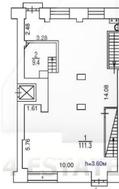
1 этаж - 123,4 кв.м.
