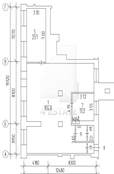
План 1 этажа после перепланировки
