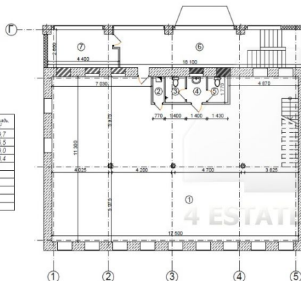
План 2-го этажа после перепланировки
