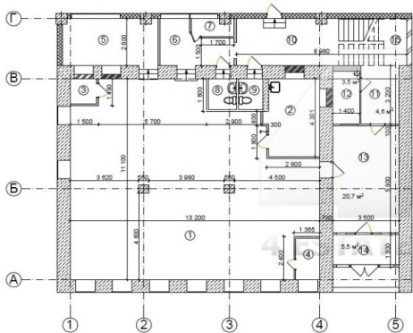
План 3-го этажа после перепланировки
