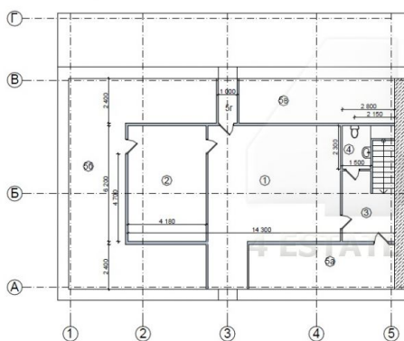
План 3-го этажа после перепланировки
