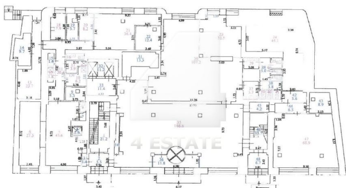
1-й этаж
